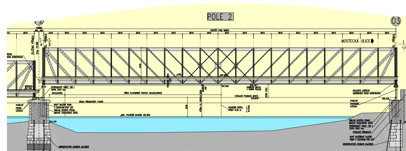
Plán pravé zdižné části Železného mostu, zdroj ŘVC ČR.
